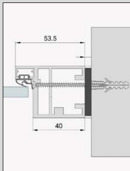
Zwischen-Wand-Montage
