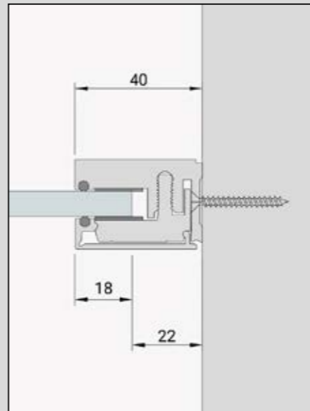
Wandanschluss-Profil
